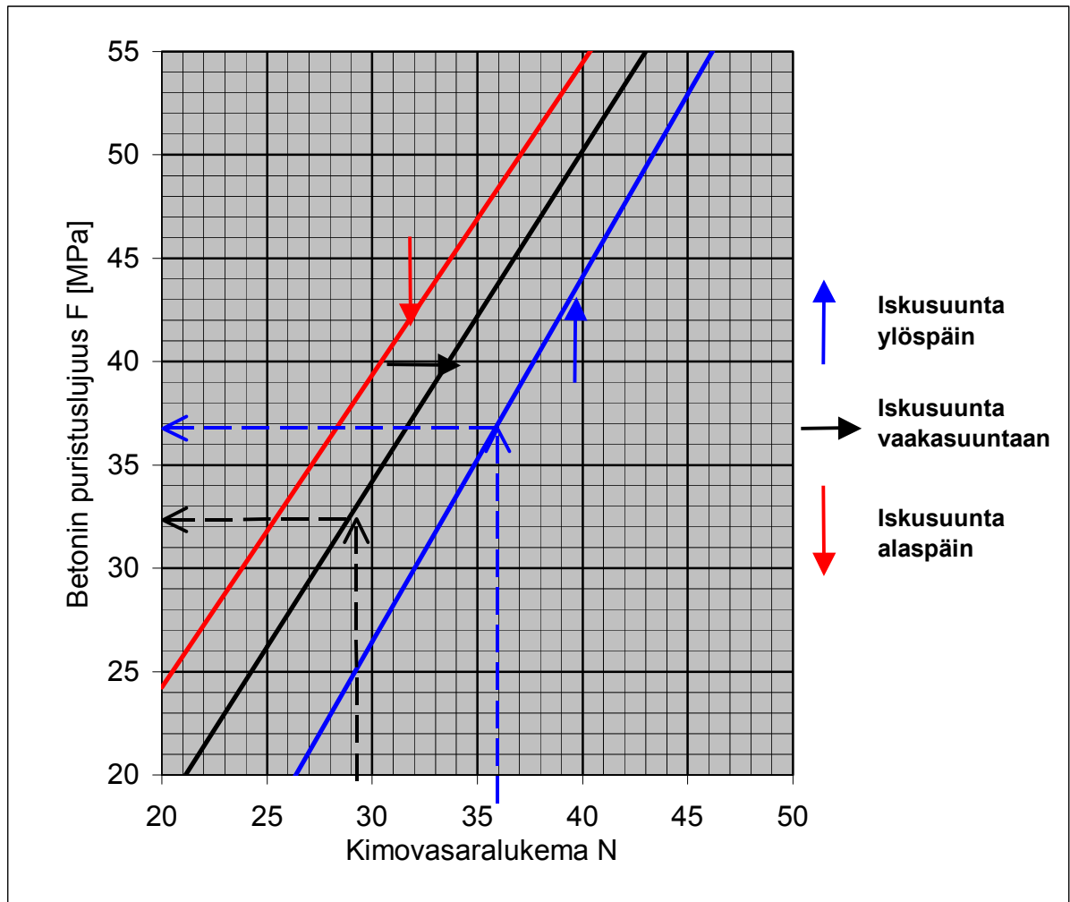
Kuva 1. Testauskohdan puristuslujuuden ja kimmovasasalukeman välinen yleinen riippuvuus.
