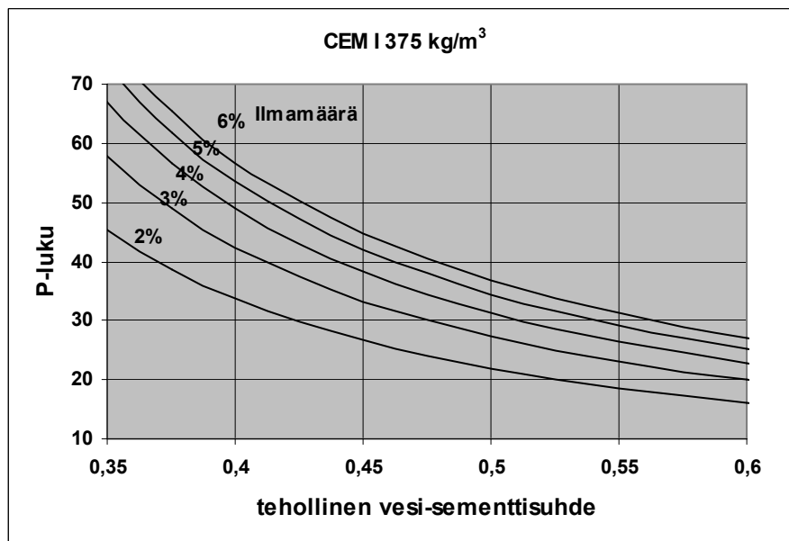
Kuva 2. Esimerkki kaavalla 1 lasketun P-luvun riippuvuudesta tehollisesta vesi-sementtisuhteesta ja ilmamäärästä sementtilaadulla CEM I sementtimäärän ollessa 375 kg/m 3 . Jälkihoitoaika 7 vuorokautta.
