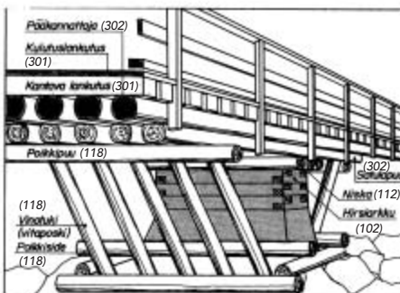
Kuva 22. Puinen tukiansassilta.
