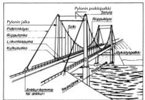
Kuva 21. Teräksinen riippusilta.
