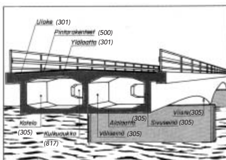
Kuva 15. Teräsbetoninen kotelopalkkisilta.
