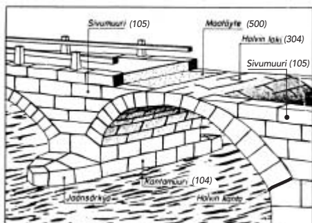
Kuva 12. Kiviholvisillan osat.
