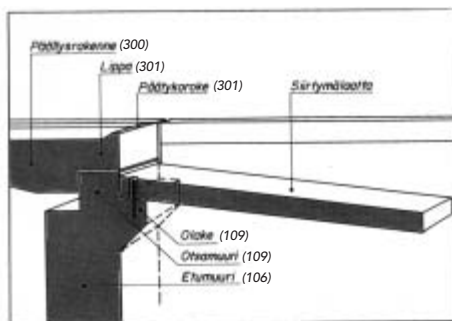
Kuva 17. Alus- ja päällysrakenteen osia sillan päässä.
