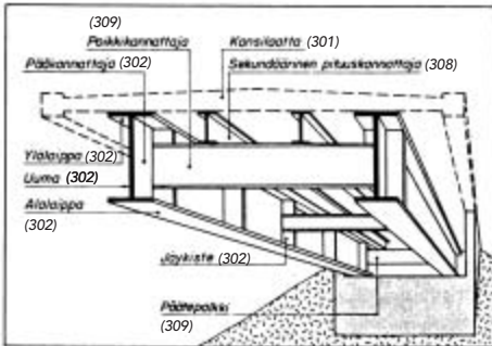
Kuva 18. Teräksinen palkkisilta.
