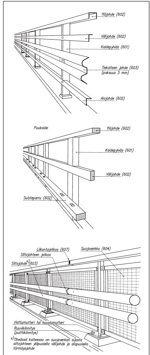
Kuva 27. Kaiteiden rakenteita.
