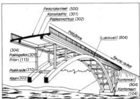
Kuva 16. Teräsbetoninen kaarisilta.
