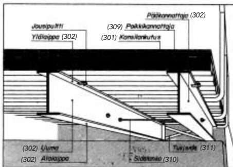
Kuva 20. Teräksinen palkkisilta, puukantinen.
