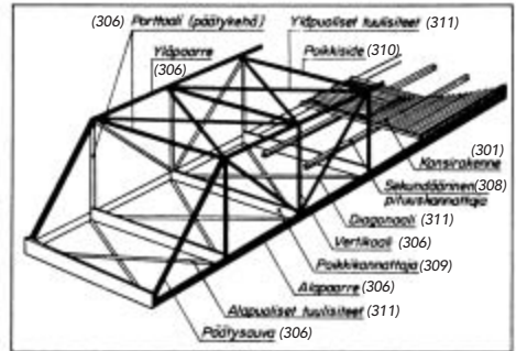
Kuva 19. Teräksinen ristikkosilta.
