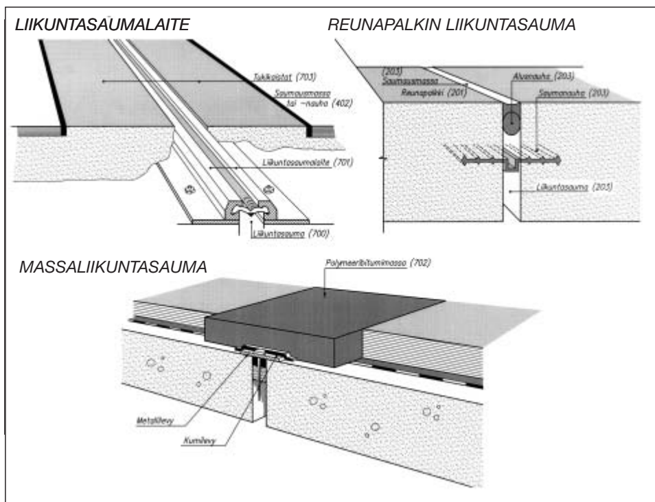
Kuva 25. Liikuntasauman rakenteita.
