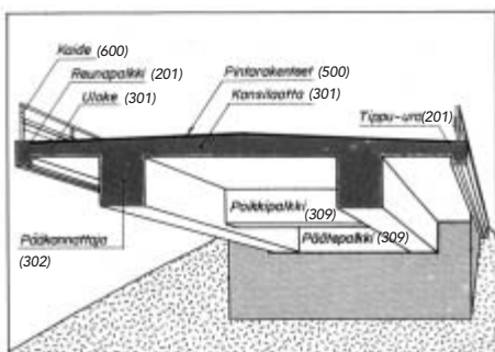
Kuva 14. Teräsbetoninen palkkisilta.
