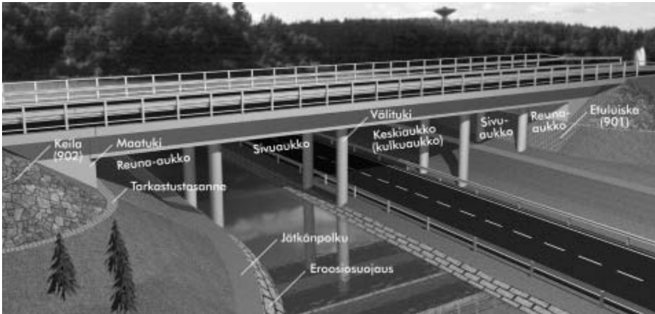
Kuva 7. Sillan alusrakenteet ja siltapaikan rakenteet.
