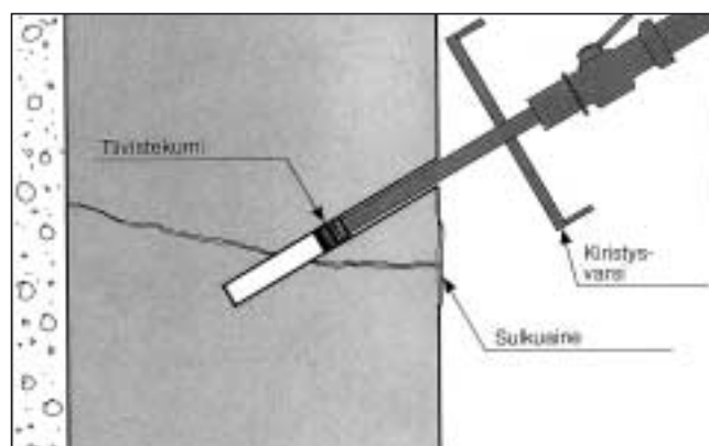
Kuva 9. Injektointitulpan kiinnitys injektointireikään.
