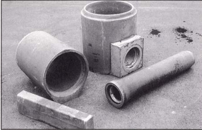
Kuva 1. Betoninen muhviputki ja uurreputki, kaivonrengas ja reunatuki.
